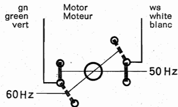
Blick von innen auf die Lötseite des Frequenzwählers bei TK 247 L
